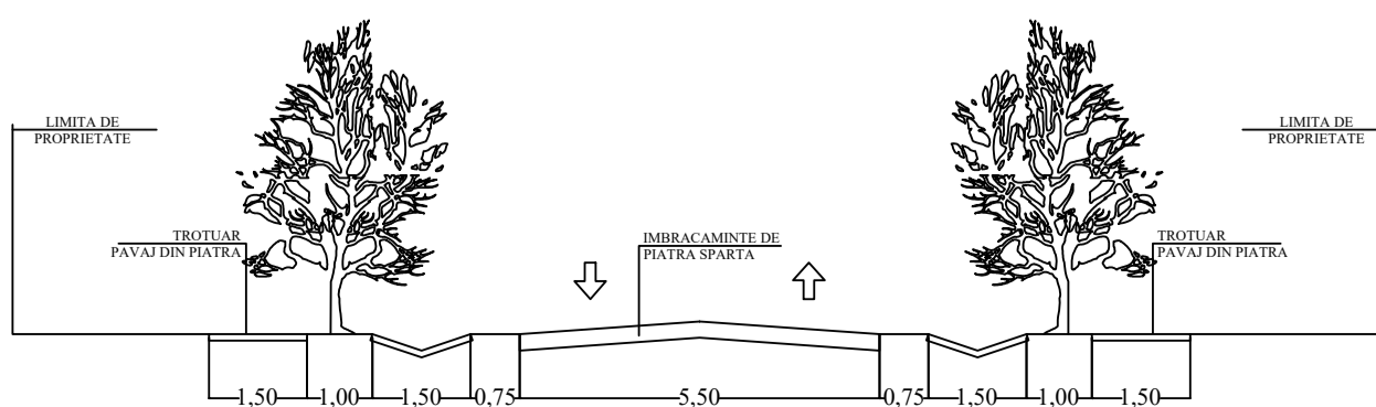
PROFIL TRANSVERSAL STRAZI, ULITE 2-2
