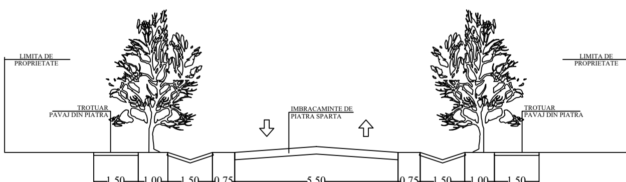
PROFIL TRANSVERSAL STRAZI, ULITE 2-2
